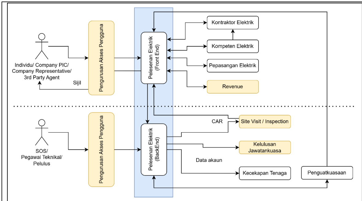
Rajah 1: Integrasi Modul LC-LE
