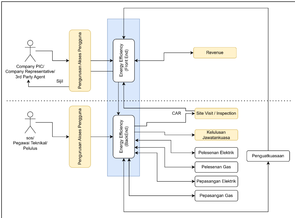
Rajah 12: Integrasi Modul EE-KT
