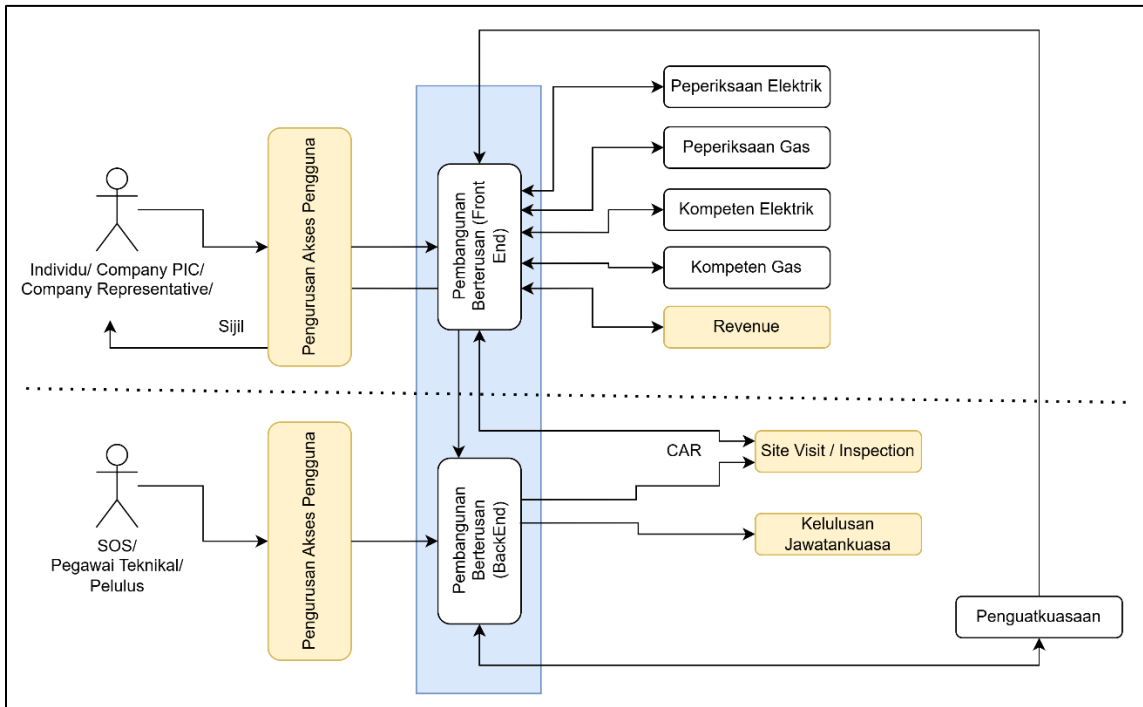
Rajah 7: Integrasi Modul CC-CD
