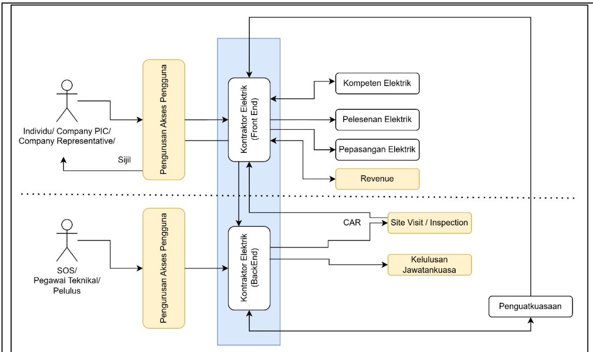
Rajah 10: Integrasi Modul RG-CE
